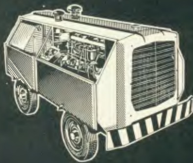
Compressor SULLAR-HOOS de parafusos helicoidais - 10,3 m 3 (365 p.c.m.)
